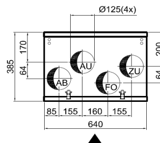
EA180.6 Bypass rechts
