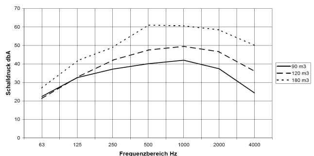
Schallwerte im Zuluftkanal -EuroAir 180
