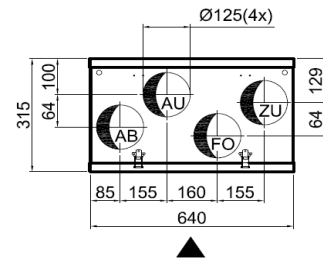
EA180.6 Basis rechts
