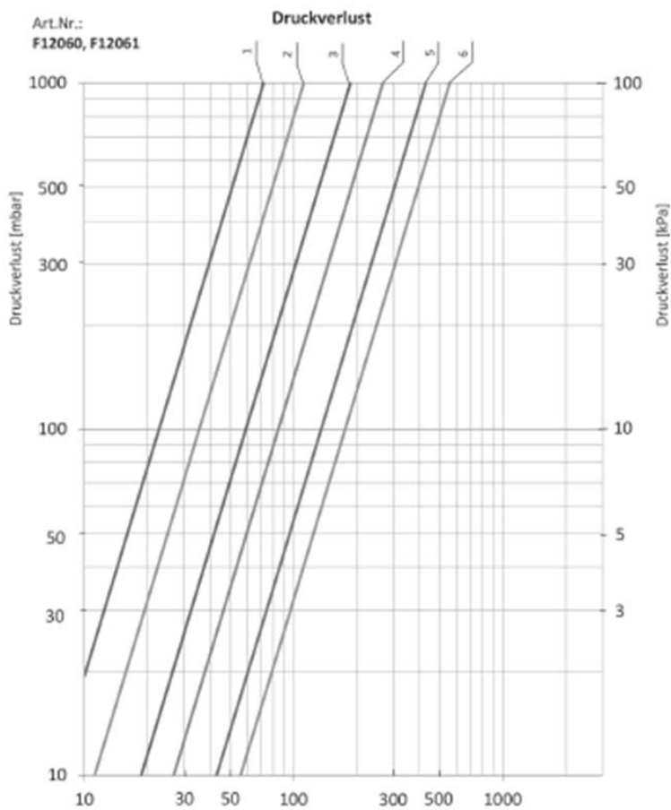
Bild 3: Druckverlustdiagramm
