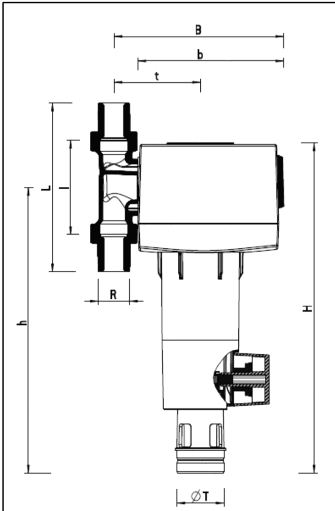
Bild 3: Baumaße Logafix Wasserfilter mit Anschlussstück
