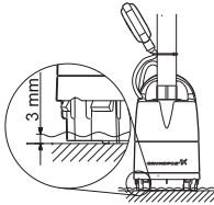
Abb. 10 Niedriger Wasserstand
