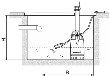
Abb. 3 Min. Einbaumaße
