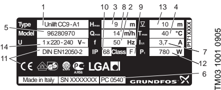
Abb. 2 Beispiel eines Leistungsschildes für Unilift CC 9
