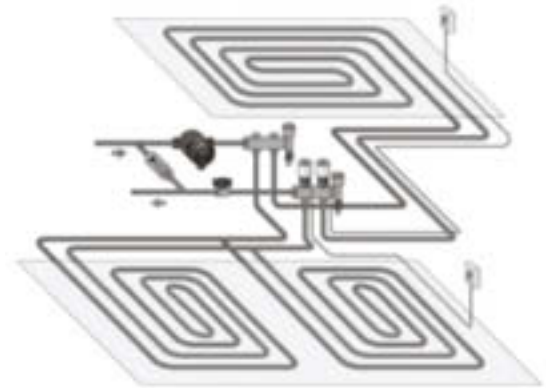
Abb. 5 Fußbodenheizung
