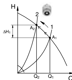
Abb. 7 Ungeregelte Pumpe
