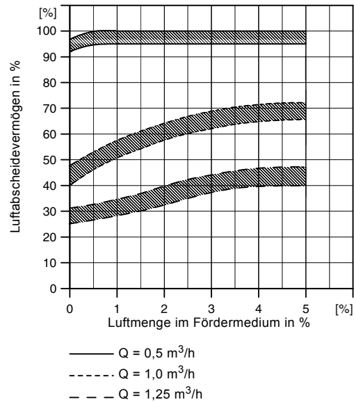
Abb. 14 Luftabscheidevermögen
