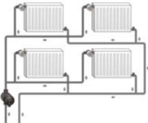
Abb. 4 Zweirohr-Heizungsanlage
