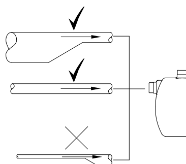
Abb. Richtige Rohrdimensionierung für den Anschluss an den Saugstutzen der Pumpe
