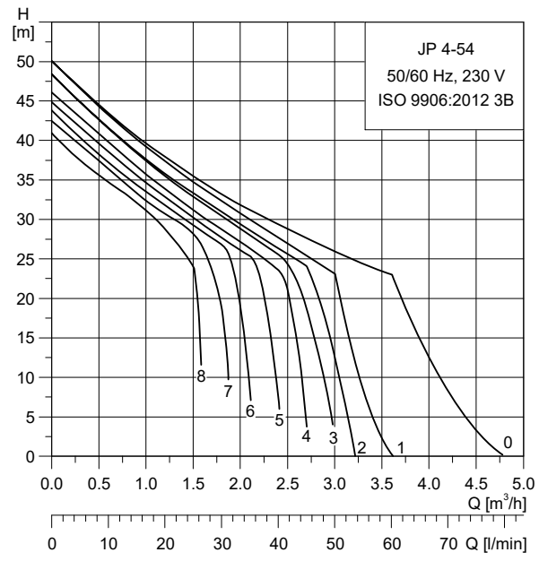
Abb. Kennlinien der JP 4-54 für Saughöhen von 0 bis 8 m
