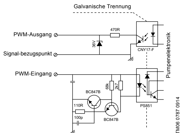
Abb. 5 Schaltplan der Schnittstelle
