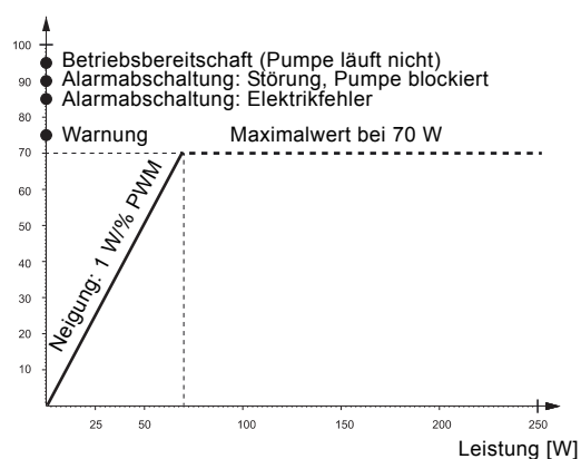
Abb. 8 PWM-Rückmeldesignal - Leistungsaufnahme
