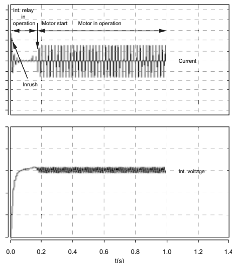
Abb. 44 Beispiel: UPM3 mit internem Einschaltstromrelais
