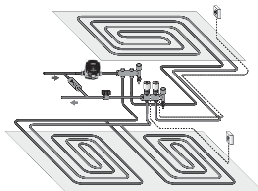
Abb. 4 Fußbodenheizung
