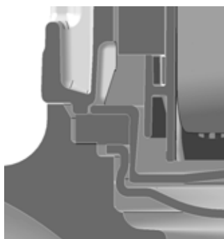
Abb. 37 Schnittzeichnung zur Veranschaulichung des Dichtungsprinzips
