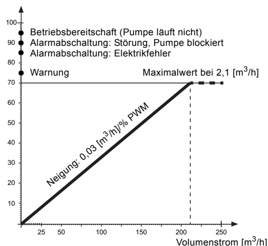
Abb. 9 PWM Rückmeldesignal - Volumenstromabschätzung
