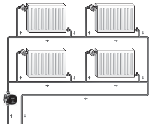
Abb. 2 Einrohrheizung
