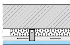
Unterdecke abgehängt mit Direktschwingabhänger D112.de
