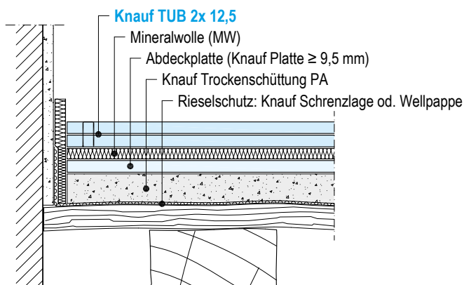
F145.de-V10 Wandanschluss Holzbalkendecke
