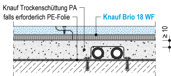
F127.de-V6 Plattenstoß
