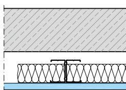
freitragende Unterdecke D131.de
