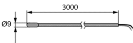
Abb. 2: Abmessungen externer Sensor des Anschluss-Sets (Angaben in mm)
