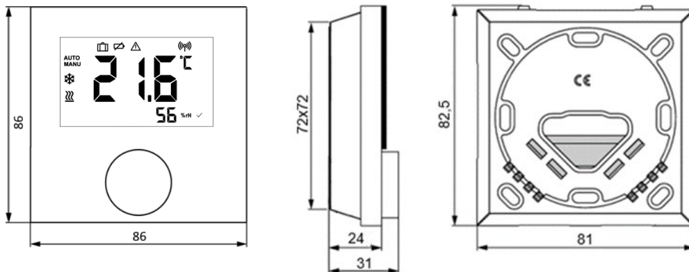
Abb. 1: Abmessungen Raumbediengerät Display (Angaben in mm)
