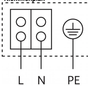
Klemmenplan
