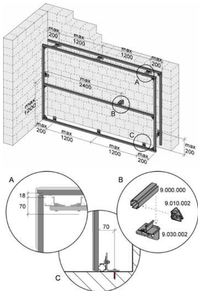
Profilwand vor einer massiven Wand
