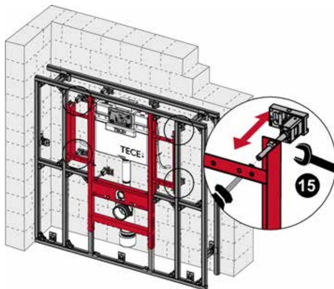
Einbau in TECEprofil Vorwand
