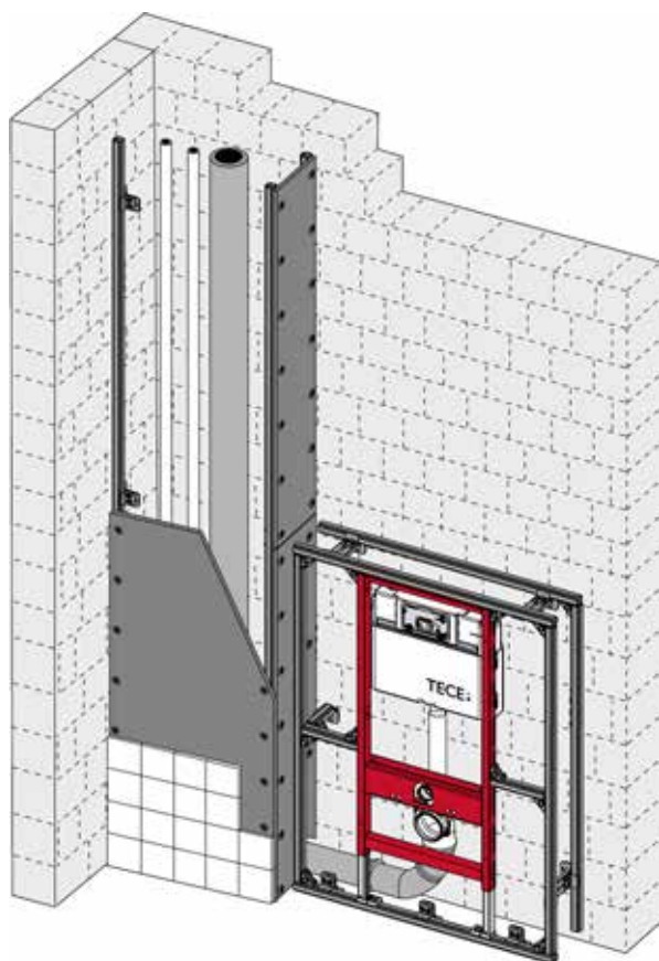
Nebenstehender Schacht, Rohrverkleidung
