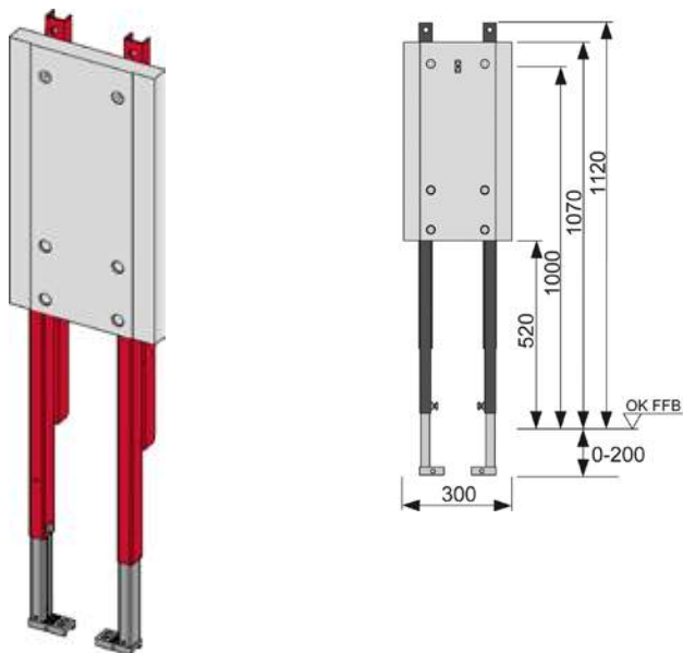
Modul für Stützgriffe und Haltesysteme (Best.-Nr. 9360000)
