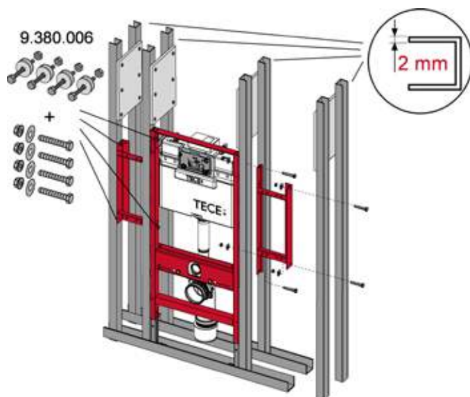
Einbau in eine Metallständerwand
