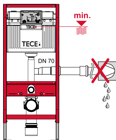
Lüfter darf nicht direkt unterhalb der Wassersäule des Spülkastens angeschlossen werden.
