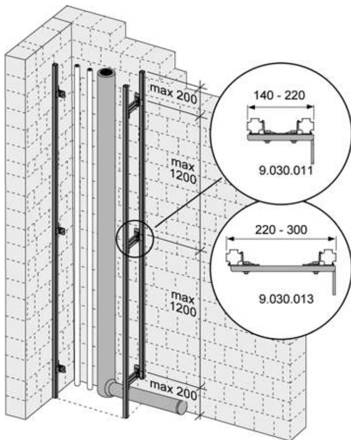
Aufgesetzter Schacht
