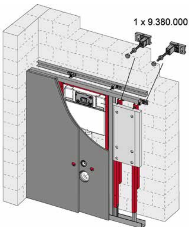
Montage des Moduls für Stützgriffe und Haltesysteme mit UA-Profil vor einer Massivwand
