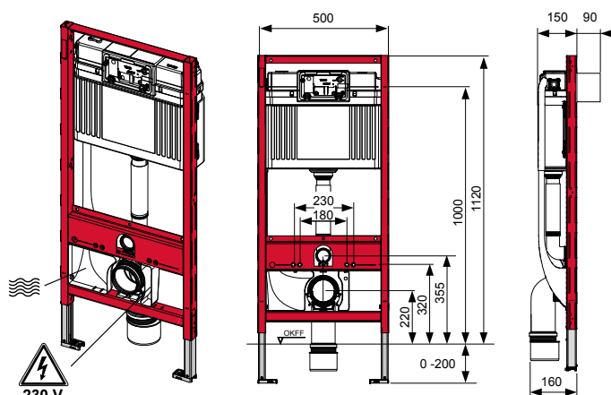
Dusch-WC-Modul 9300079
