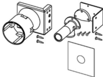
Aufrüstset für wandhängende Dusch-WC-Aufsätze (Best.-Nr. 9880037)
