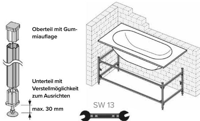
Einbau einer Stahlwanne in ein TECEprofil Tragegerüst
