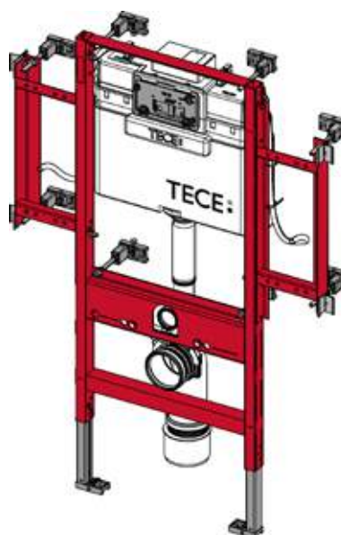
TECE-Gerontomodul (Best.-Nr. 9300009)
