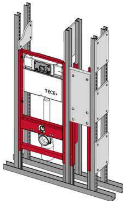
Montage des Moduls für Stützgriffe und Haltesysteme in eine frei stehende Wand mit UA-Profil
