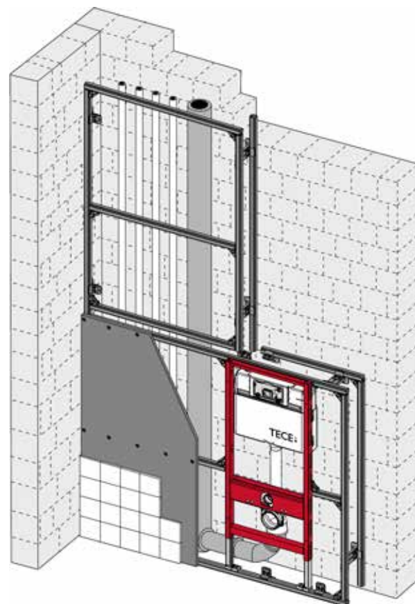
Aufgesetzter Schacht
