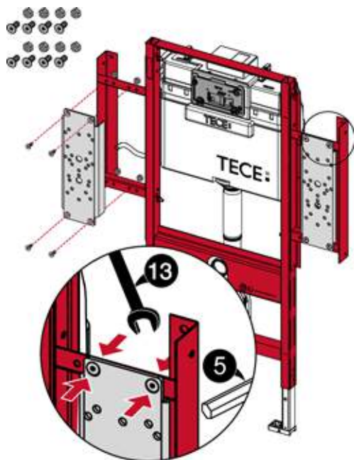
Montage der seitlichen Stahlplatten an das Gerontomodul
