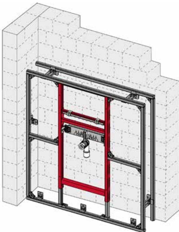
Modulbauweise mit Universalmodul für Waschtisch
