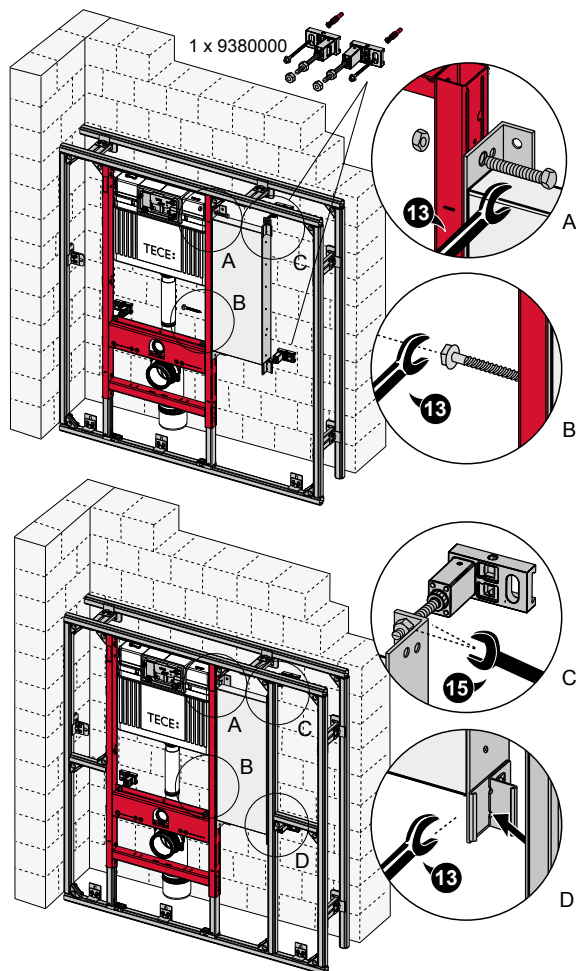
Montage der Befestigungsplatte für Stützklappgriffe mit Wandbefestigung (oben) bzw. Multiklemmen und Profilrohr (unten)
