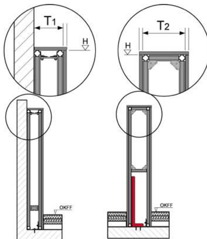
Mögliche Vorwandhöhen mit TECEprofil Tragwerk - 2
