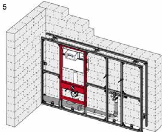
Waagerechte Mittelstreben montieren
