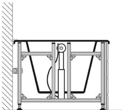
TECEprofil Tragwerk beim Einbau einer Überlaufgarnitur
