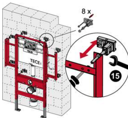
Einbau als Einzelmodul vor einer Massivwand
