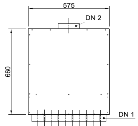
Draufsicht
