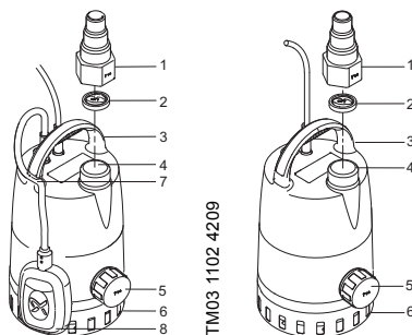
Abb. 1 Pumpen mit und ohne Schwimmerschalter
