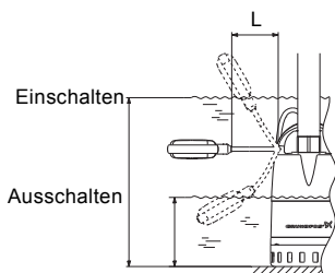
Abb. 9 Ein-/Ausschaltniveau bei mind. und max. Kabellängen
